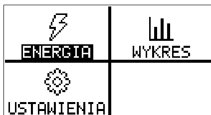
Rys. 8.9. Menu główne
